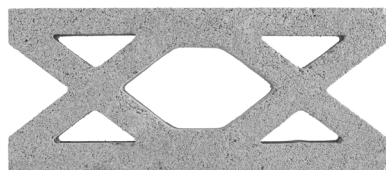
VISTA 4 x 8 x 18 | 22 LBS 39% VOID PER UNIT
