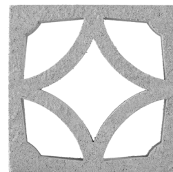
CORDOVA 4 x 12 x 12 | 22 LBS 39% VOID PER UNIT
