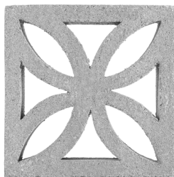
LA COSTA 4 x 12 x 12 | 24 LBS 33% VOID PER UNIT
